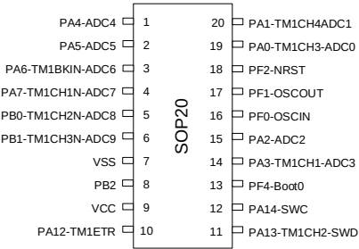
图 3-6 SOP20 Pinout1 PY32F003F1xS
