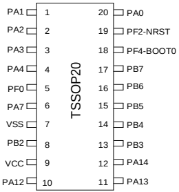
图 3-4 TSSOP20 Pinout3 PY32F003F3xP
