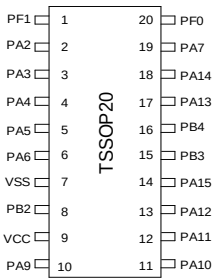
图 3-5 TSSOP20 Pinout4 PY32F003F4xP
